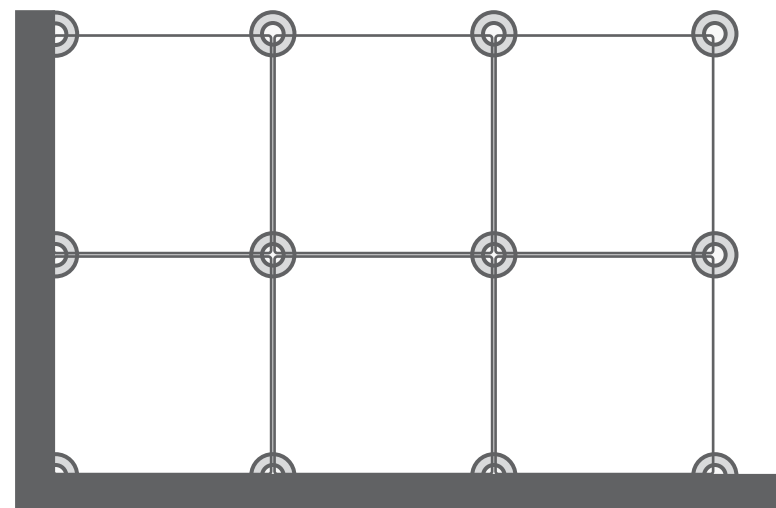
Przykładowy schemat ułożenia płyt 60x60 na wspornikach.
